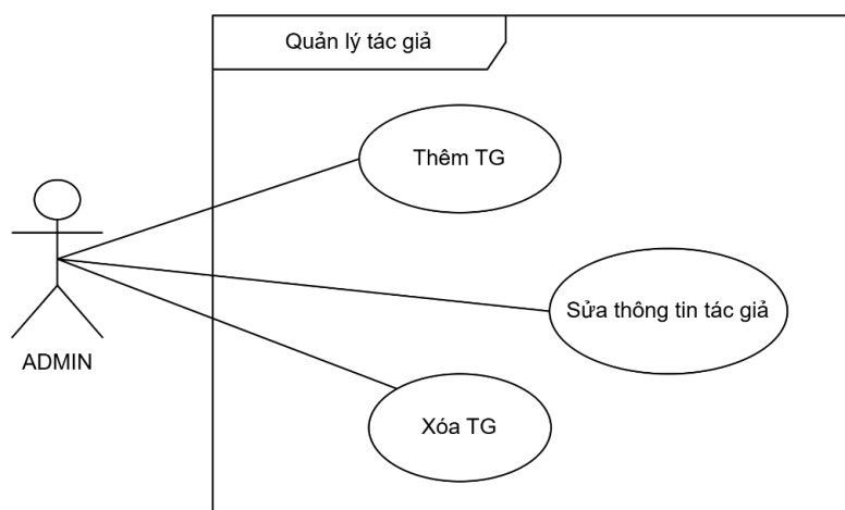
Hình 1.7: Biểu đồ phân rã UC QL TG
