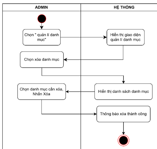
Hình 1.15: Biểu đồ hoạt động xóa danh mục
