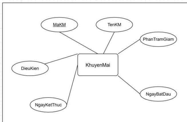
Hình 2.15: Mô hình chi tiết thực thể KhuyenMai
