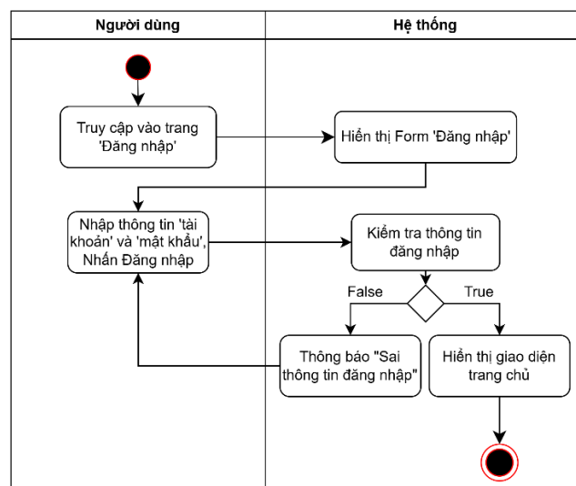
Hình 1.8: Biểu đồ hoạt động Đăng nhập tài khoản
