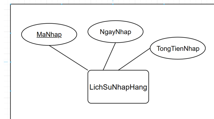
Hình 2.11: Mô hình chi tiết thực thể LichSuNhapHang
