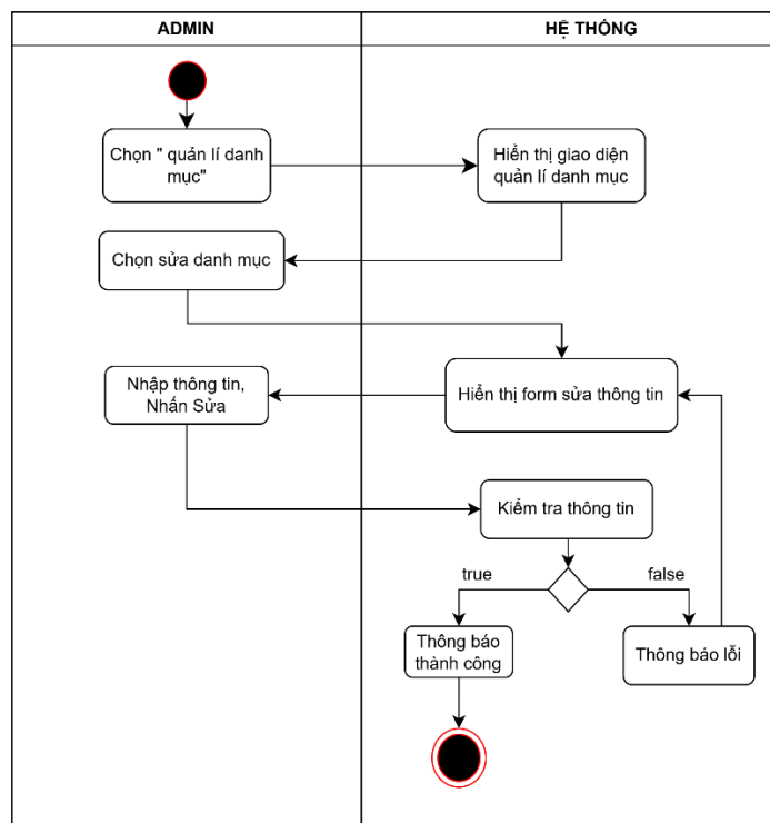
Hình 1.14: Biểu đồ hoạt động Sửa danh mục
