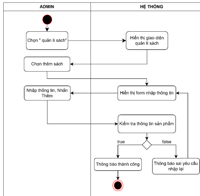
Hình 1.10: Biểu đồ hoạt động Thêm sách
