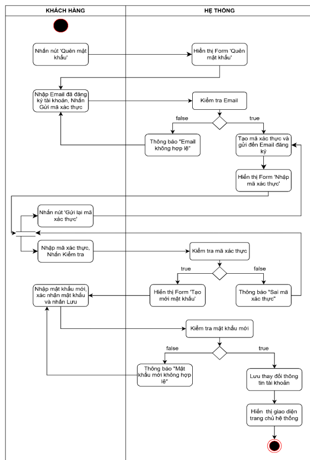
Hình 1.16: Biểu đồ hoạt động Quên mật khẩu
