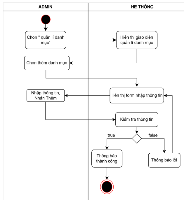
Hình 1.13: Biểu đồ hoạt động Thêm danh mục
