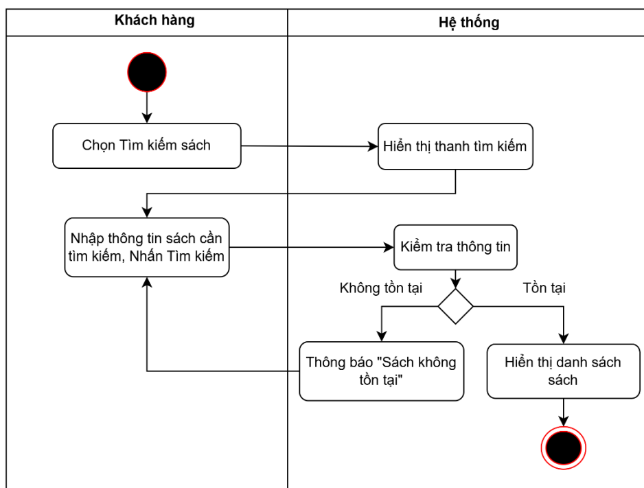
Hình 1.17: Biểu đồ hoạt động tìm kiếm sách
