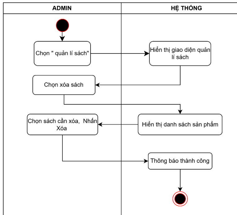
Hình 1.11: Biểu đồ hoạt động Xóa sách
