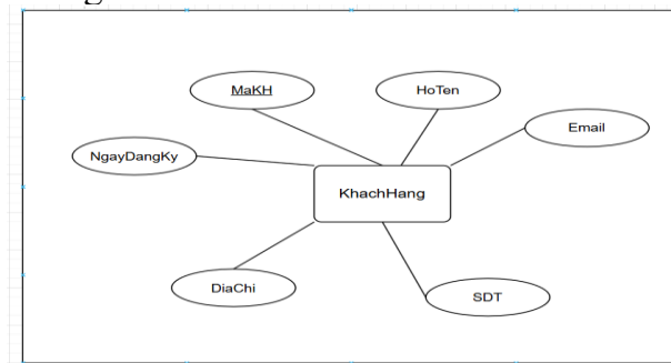
Hình 2.5: Mô hình chi tiết thực thể KháchHàng
