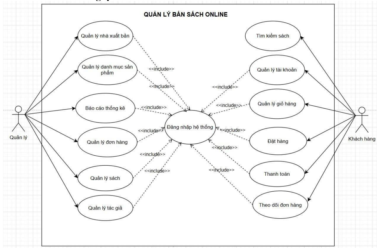
Hình 1.1 : biểu đồ UC tổng quát
