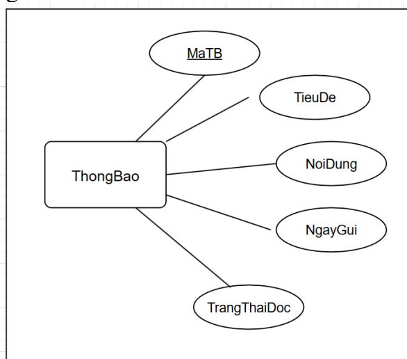
Hình 2.16: Mô hình chi tiết thực thể ThôngBao
