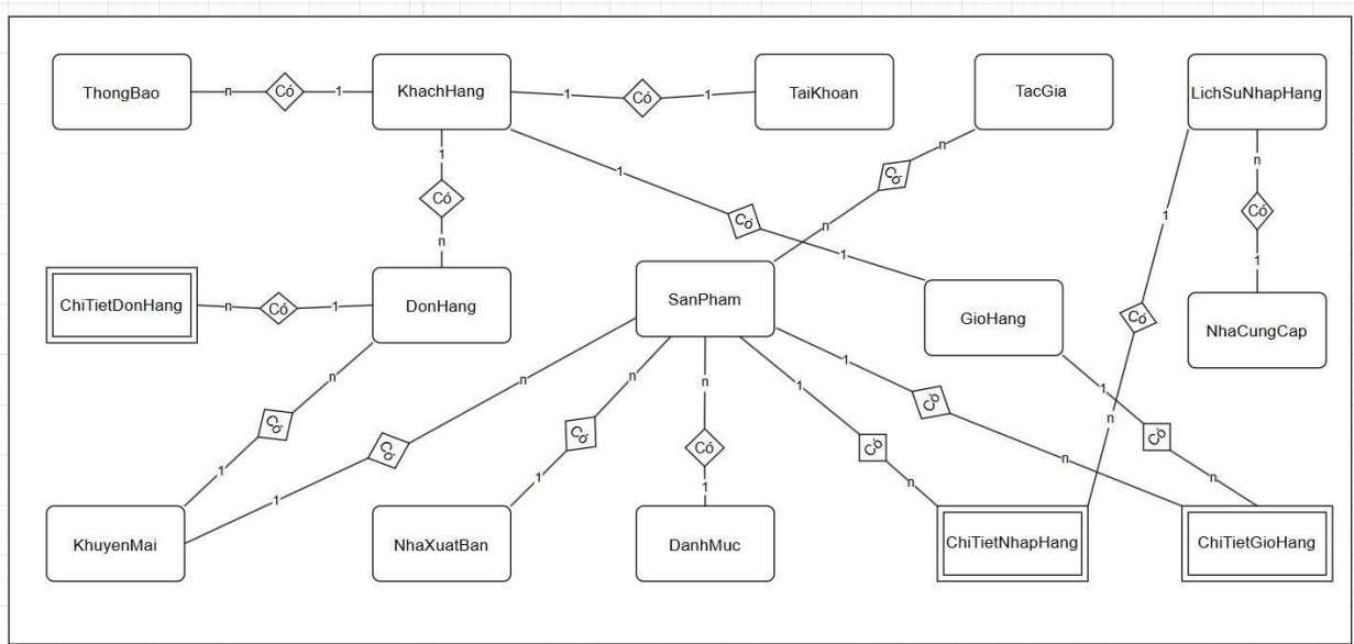
Hình 2.3 : Mô hình thực thể liên kết
