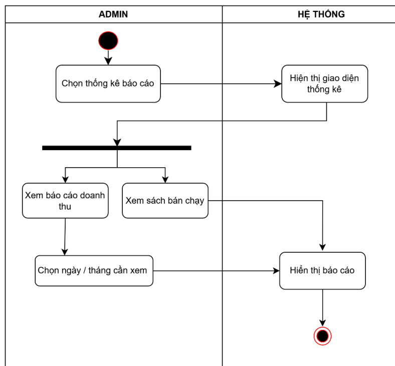
Hình 1.20: Biểu đồ hoạt động thống kê báo cáo
