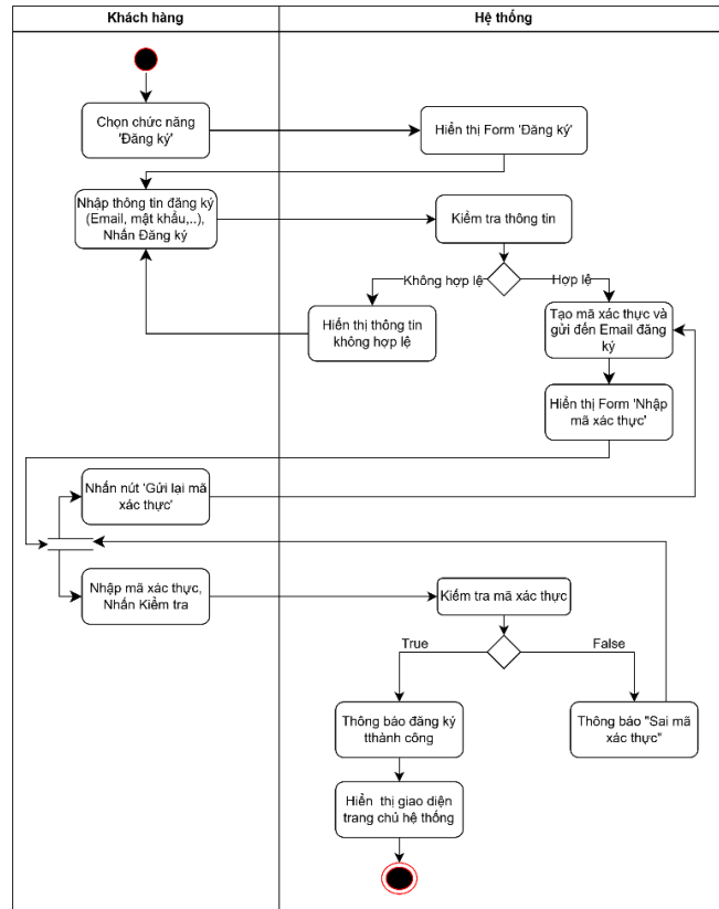
Hình 1.9: Biểu đồ hoạt động Đăng ký tài khoản
