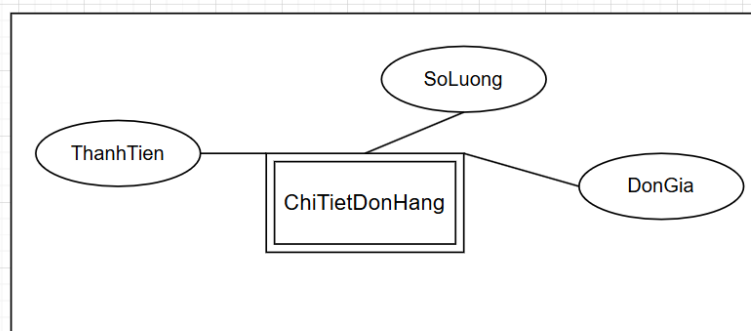
Hình 2.10: Mô hình chi tiết thực thể ChiTietDonHang
