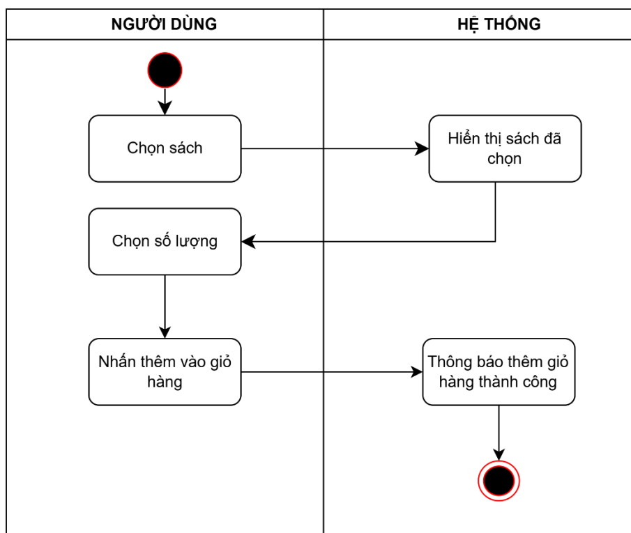
Hình 1.18: Biểu đồ hoạt động thêm sách vào giỏ hàng
