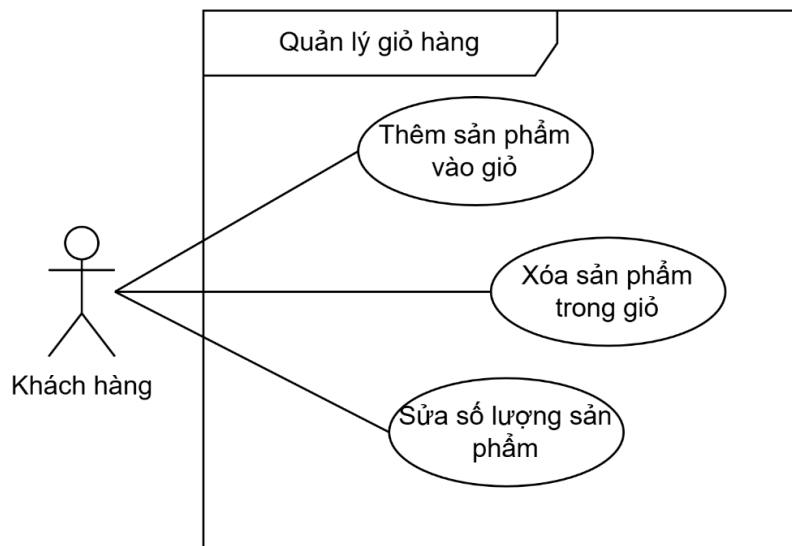
Hình 1.6: Biểu đồ phân rã UC QL giỏ hàng
