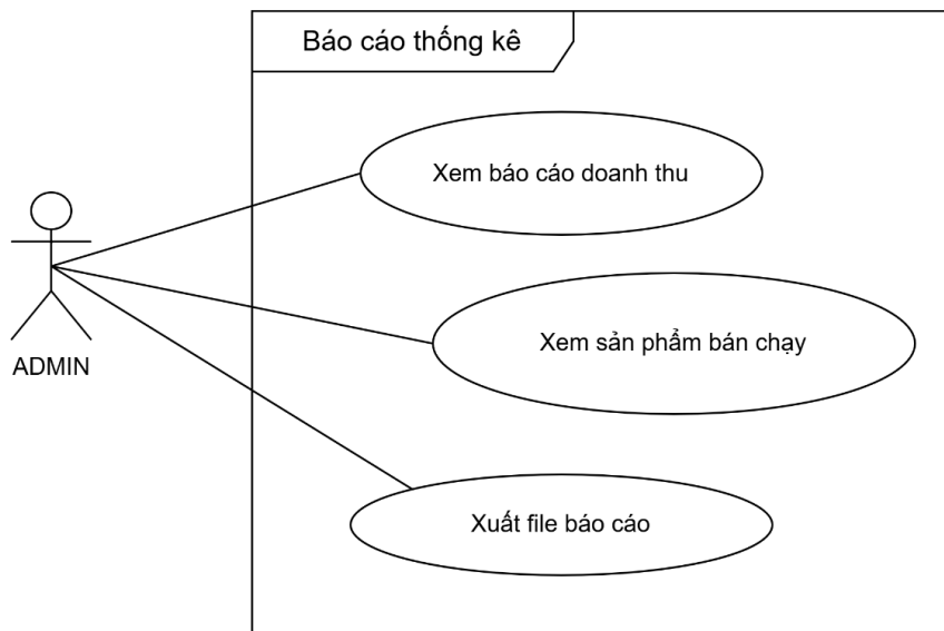
Hình 1.4: Biểu đồ phân rã UC BCTK
