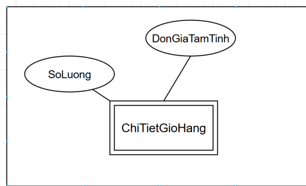
Hình 2.14: Mô hình chi tiết thực thể ChiTietGioHang
