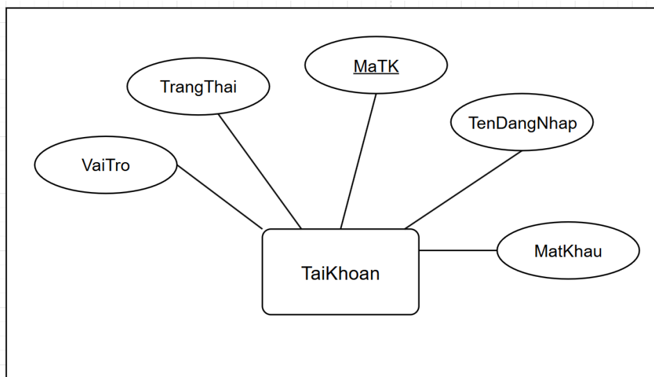
Hình 2.4: Mô hình chi tiết thực thể TàiKhoan
