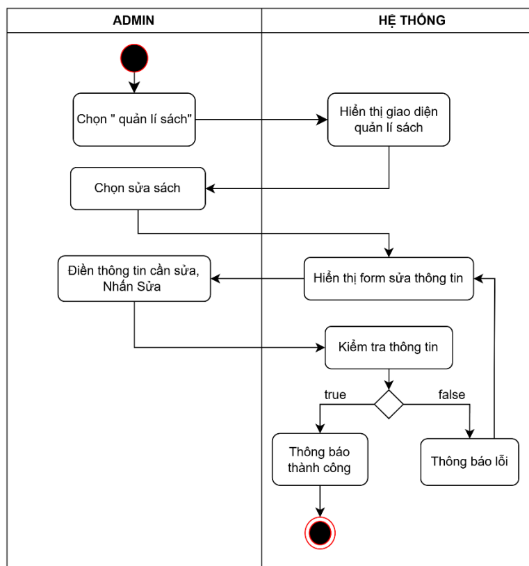
Hình 1.12: Biểu đồ hoạt động Sửa sách
