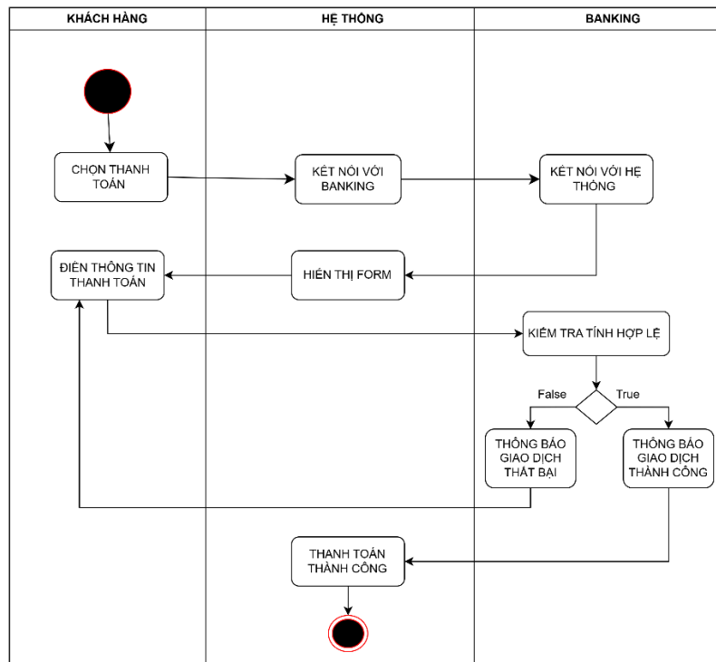
Hình 1.19: Biểu đồ hoạt động thanh toán
